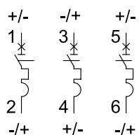
3P (6kA) or (10kA)
