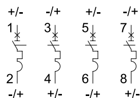
4P (6kA) or (10kA)
