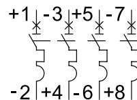
4P (6kA) or (10kA)
